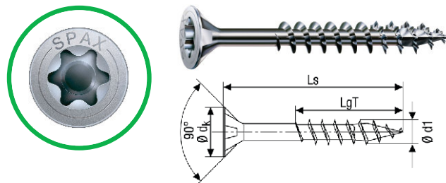
SPAX T-STAR GLAVA - DELIMIČAN NAVOJ
