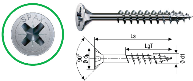
SPAX PZ GLAVA - DELIMIČAN NAVOJ
