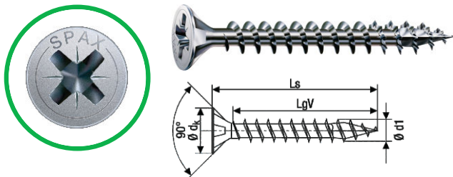
SPAX PZ GLAVA - PUN NAVOJ
