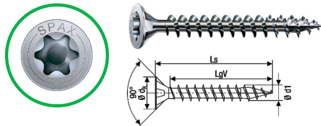
SPAX T-STAR GLAVA - PUN NAVOJ
