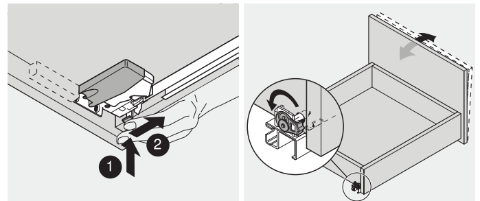
Podešavanje visine +3 mm
