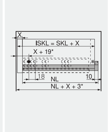
ISKL Unutrašnja dužina fioke SKL Dužina fioke NL Nominalna dužina
