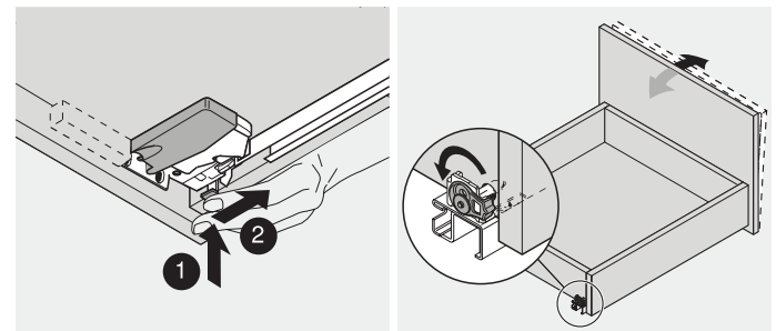
Podešavanje visine +3 mm
