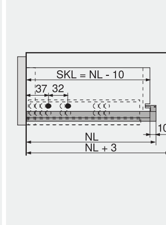
SKL Dužina fioke NL Nominalna dužina
