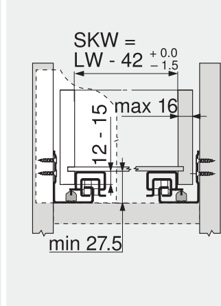
SKW Unutrašnja širina fioke LW Unutrašnja širina korpusa
